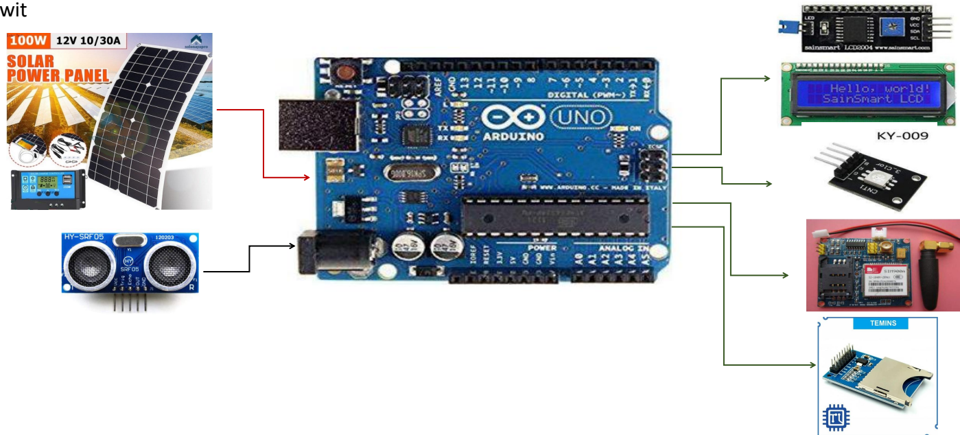
Gambar 2. Skematik pengembangan rangkaian alat pemantau dan pemberi peringatan tinggi muka air lahan gambut (catu daya, input sensor, mikrokontroler, dan 4 jenis output )
