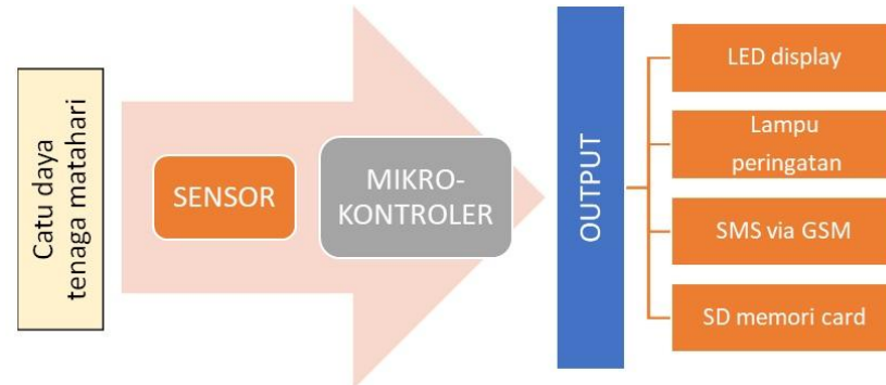
Gambar 1. Bagan kerangka fungsional setiap komponen alat pemantau dan pemberi peringatan tinggi muka air kritis lahan gambut kelapa sawit
