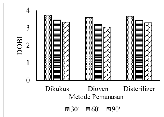
Gambar 2. Hubungan metode dan waktu pemanasan terhadap nilai DOBI minyak sawit
