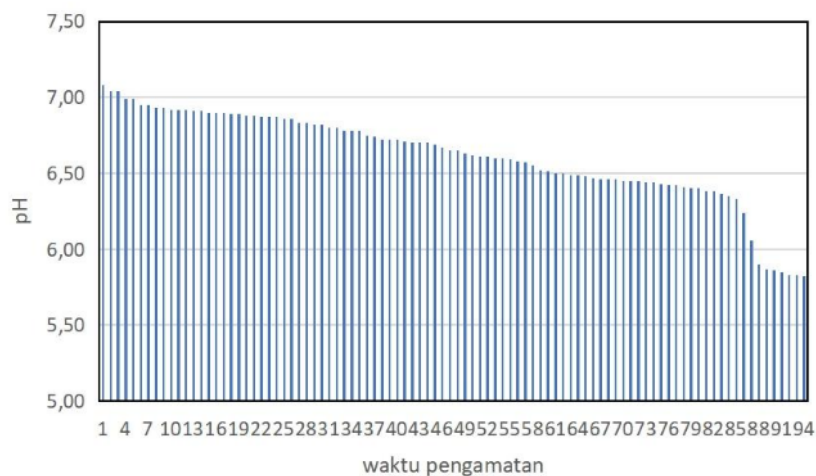
Gambar 10. Hasil pengukuran tingkat keasaman (pH) nira oleh SPVAN saat penyadapan dari pukul 07.00 - 15.30
