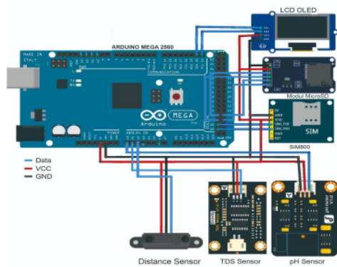
Gambar 5. Skema rangkaian elektronik perangkat pemantau volume dan keasaman nira berbasis mikrokontroler
