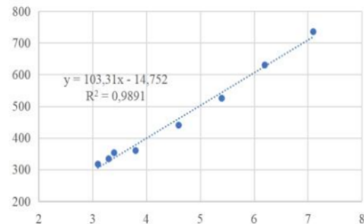
Gambar 9. Hubungan Antara Pembacaan Tegangan Sensor dengan Nilai pH
